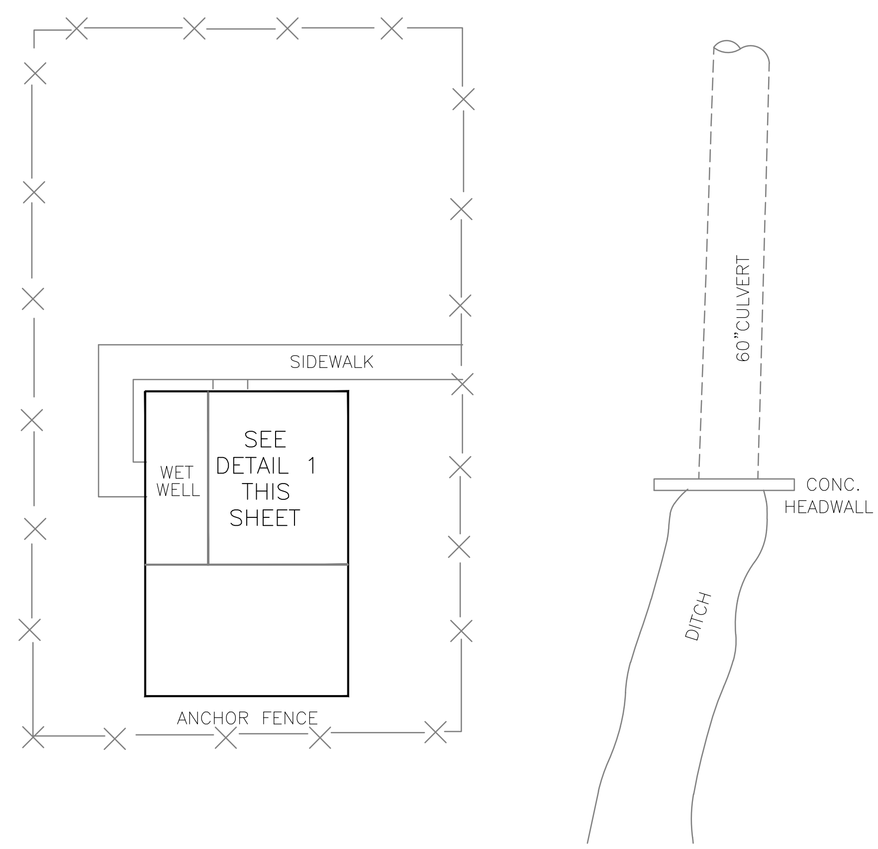
5 SITE PLAN SCALE: 1/8" = 1'-0"
